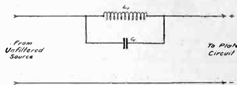
Fig. 7. Trap Circuit.
