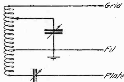
FIG. 1 Hartley-Reinartz
